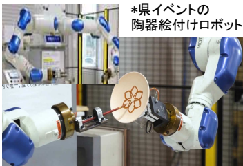
安川電機 DIA10 15軸双腕(組立)ロボット
