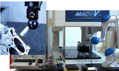
ミツビシ MACH9106 インライン対応CNC3次元自動測定ロボットシステム(国際ロボット展2017展示機)
